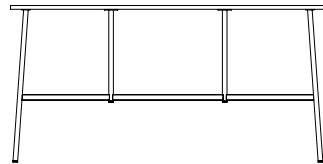
Union Bar Table 190 x 90 cm x H95,5 cm H: 95,5 x L: 190 x D: 90 cm
